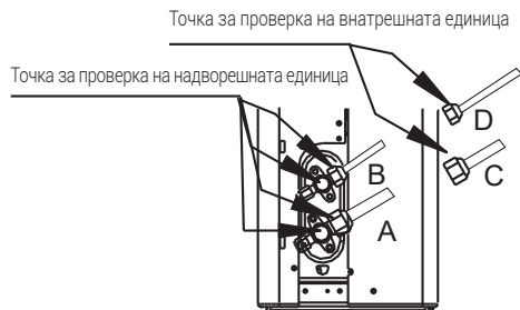
A: Стоп-вентил за низок притисок B: Стоп-вентил за висок притисок C и D: Навртки за проширување на внатрешната единица
